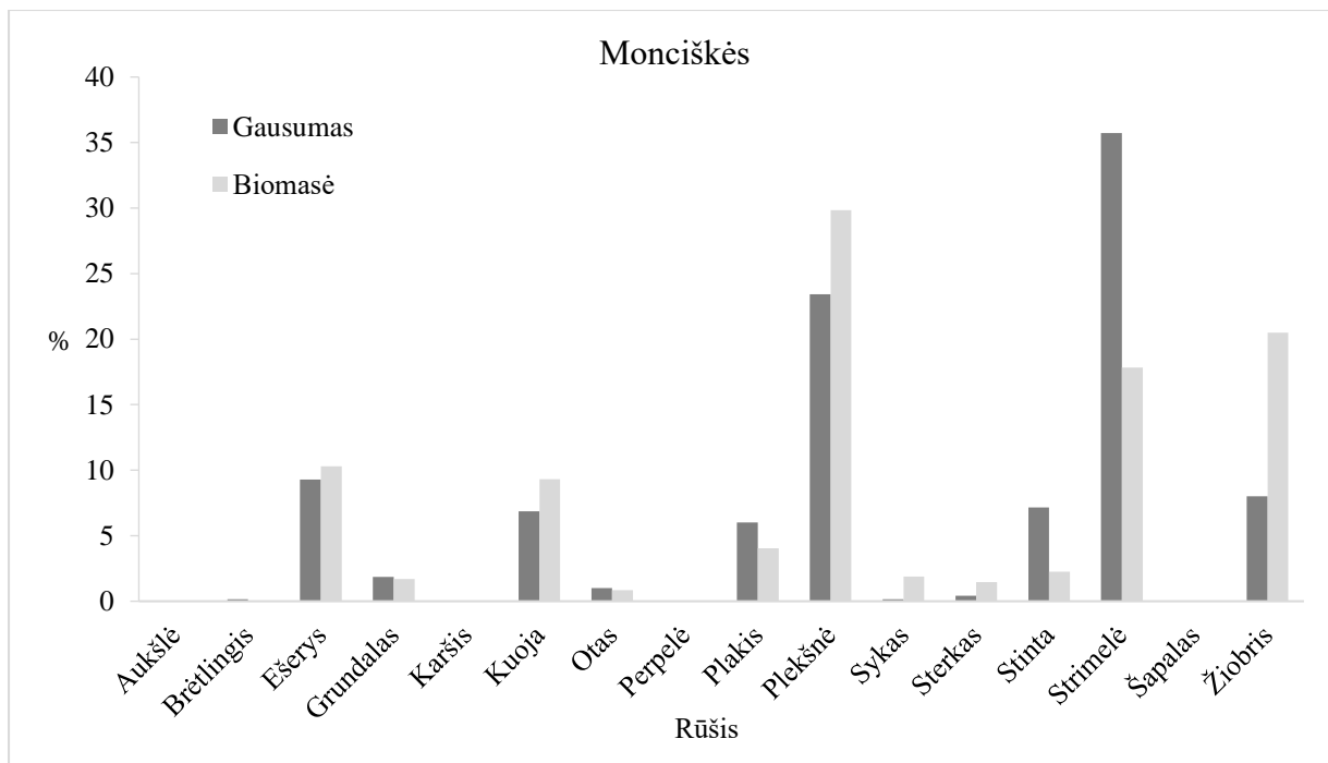
2.6 pav. Žuvų bendrijos sudėtis pagal gausumą ir pagal biomasę akvatorijoje ties Mončiškėmis 2019 m.
