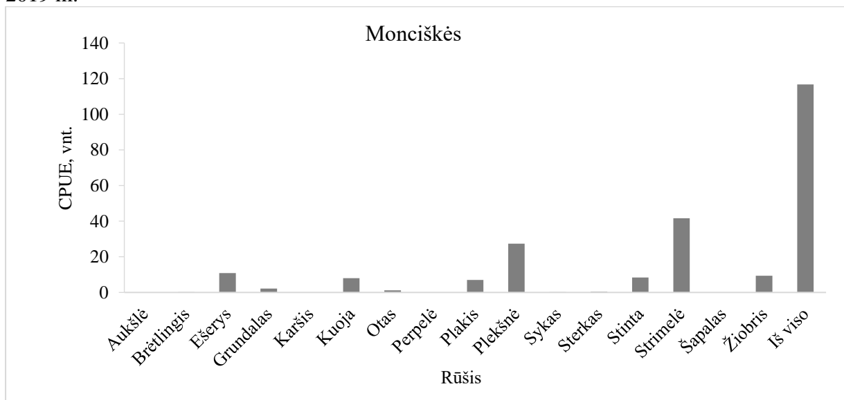
2.7 pav. Žuvų sugavimai vienai standartinei žvejybos pastangai (CPUE) akvatorijoje ties Mončiškėmis 2019 m.
