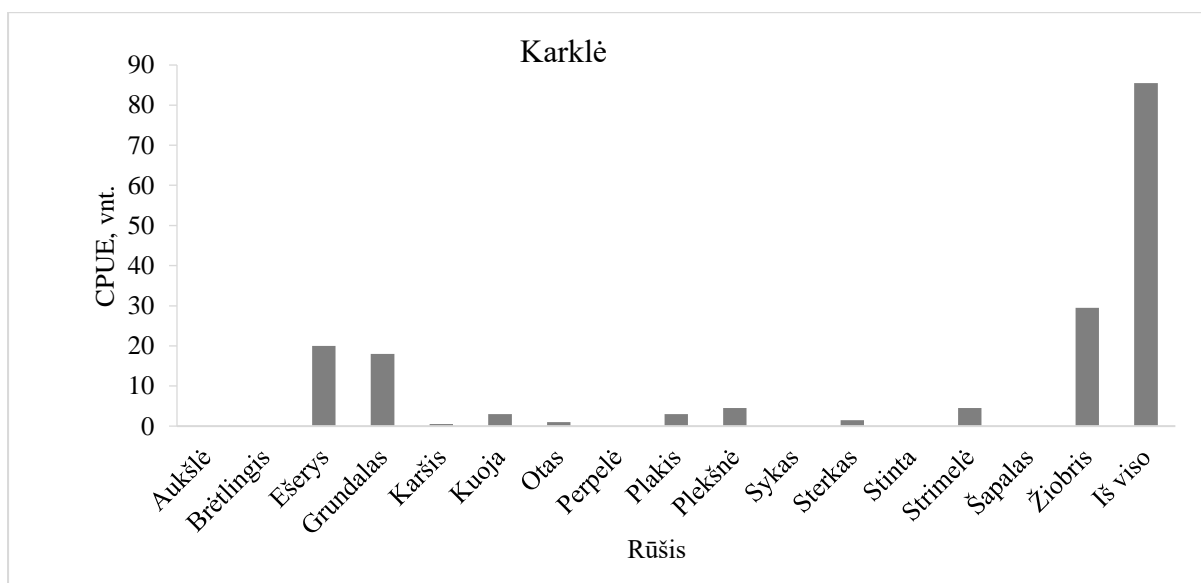
2.11 pav. Žuvų sugavimai vienai standartinei žvejybos pastangai (CPUE) akvatorijoje ties Karkle 2019 m.
