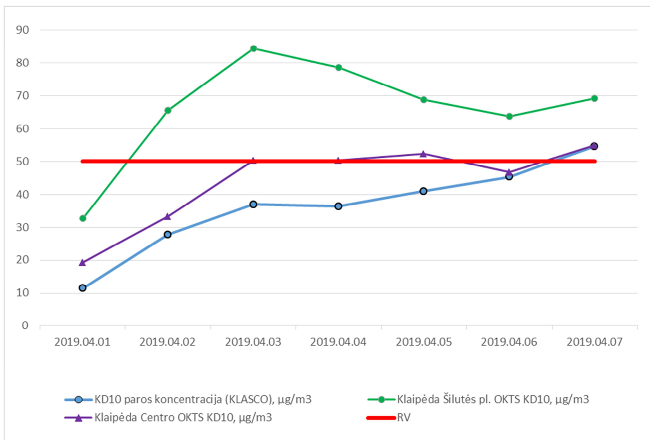
1 pav. Vidutinė paros KD_{10} koncentracija KLASCO teritorijoje N.Uosto g. 23 ir Klaipėdos oro kokybės tyrimų stotyse
